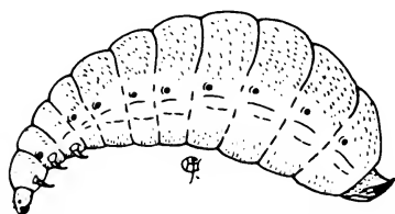
Fig. 238. Sandalus niger Knoch.
